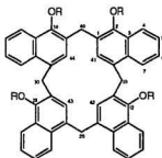
10 R=H 10a R=Bz 10b R=Ac
