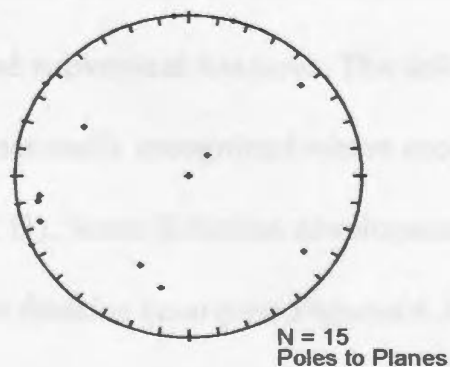
E. Faults
