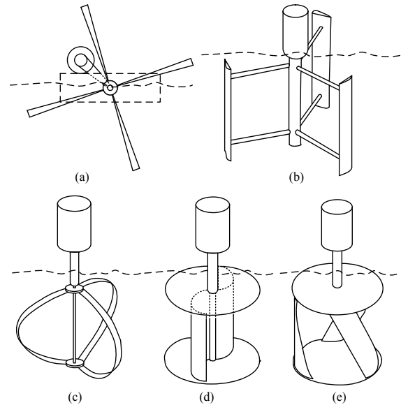
Fig. 3. Cross flow turbines (a) In-plane (b) H-Darrieus (c) Darrieus (d) Savonius (e) Helical
